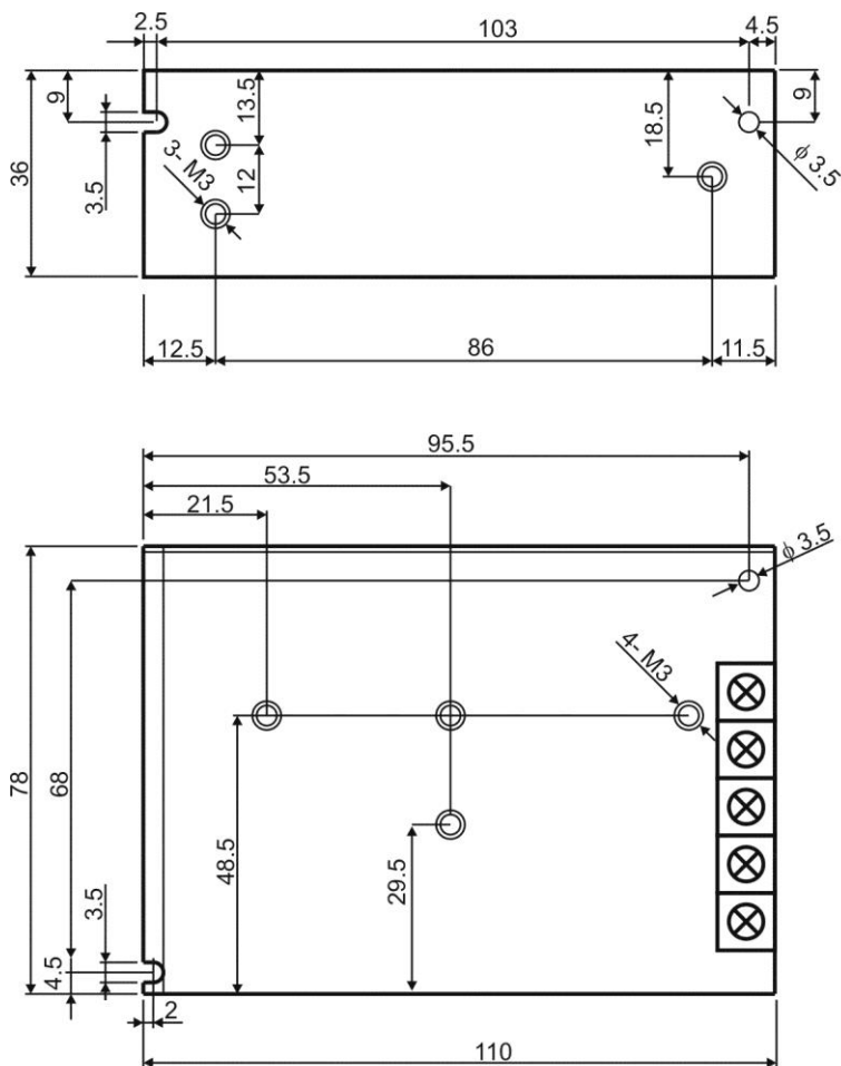
Rysunek 2. Widok mechaniczny zasilacza
